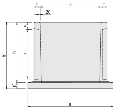
側面図 (1)
