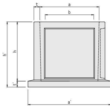
側面図 (2)
